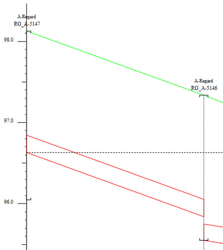
Figure 130 : Tracé d'un linéaire utilisant ses côtés fil d'eau
