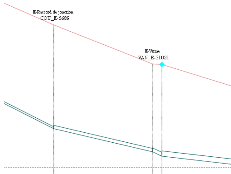
Figure 108 : Exemple tracé des ponctuels en extrémité
