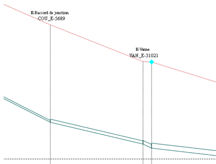
Figure 111 : Exemple d'un tracé de ponctuels d'extrémité (Eau)
